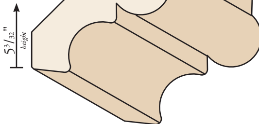
20M232-CR 20mm x 7\frac{1}{4} " (45°)
